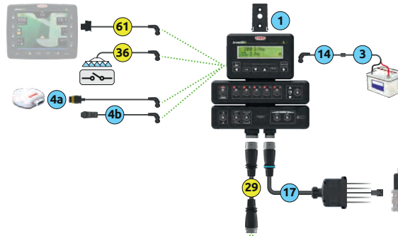
SCHEMA DI INSTALLAZIONE SCHÉMA D'INSTALLATION INSTALLATIONSPLAN
